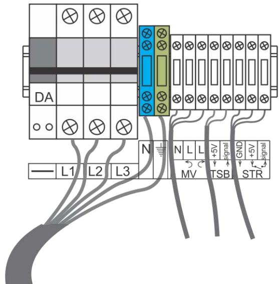
Afbeelding 9c: NOARK zekeringen
